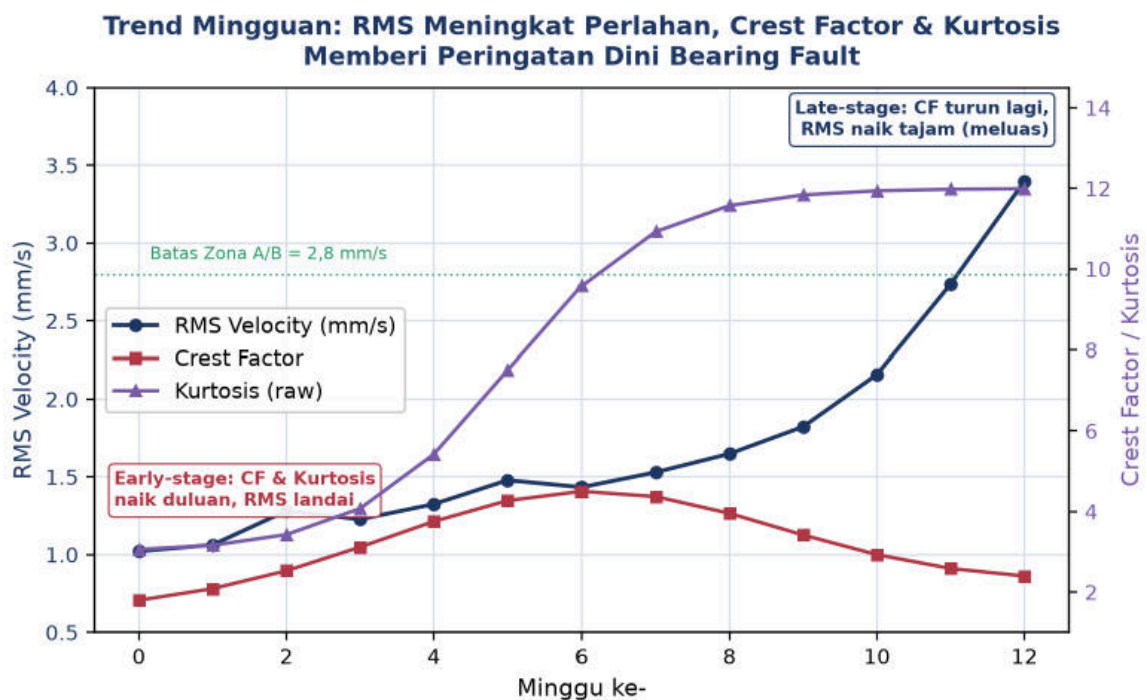
Gambar 6 Trend ming g uan RMS, Crest Factor, dan Kurtosis pada prog resi kerusakan bearing : CF dan Kurtosis naik lebih dulu (early-stage), RMS naik tajam belakangan (late-stage), sementara CF justru turun kembali saat kerusakan meluas.
