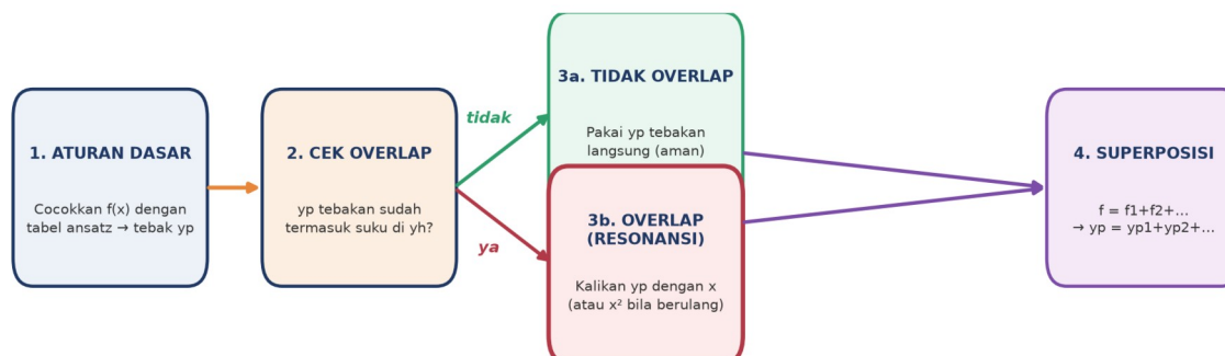
Gambar 2. Diagram alir tiga aturan penentuan yp pada metode Koefisien Tak Tentu: aturan dasar, cek overlap dengan y_h (resonansi), dan superposisi.
