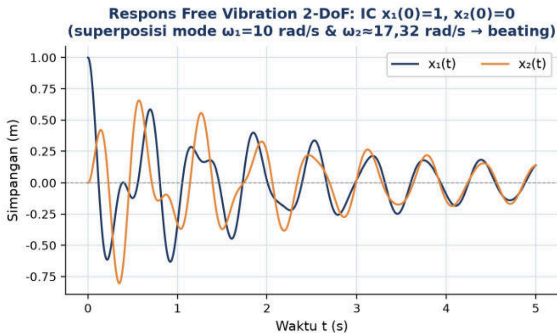
Gambar 6. Respons free vibration sistem referensi 2-DoF hasil solve_ivp initial condition x_1(0)=1 , \dot{x}_1(0)=0 , menunjukkan pola beating dari superposisi dua mode.
