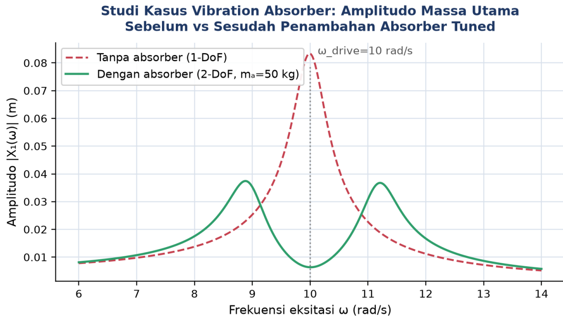
Gambar 6. Studi kasus vibration absorber: kurva amplitudo massa utama sebelum (garis putus merah, resonansi tunggal di \omega_{drive}=10 rad/s) dan sesudah penambahan absorber tuned (garis hijau, anti-resonansi di \omega_{drive} dengan dua puncak baru mengapit di 8,94 dan 11,18 rad/s).
