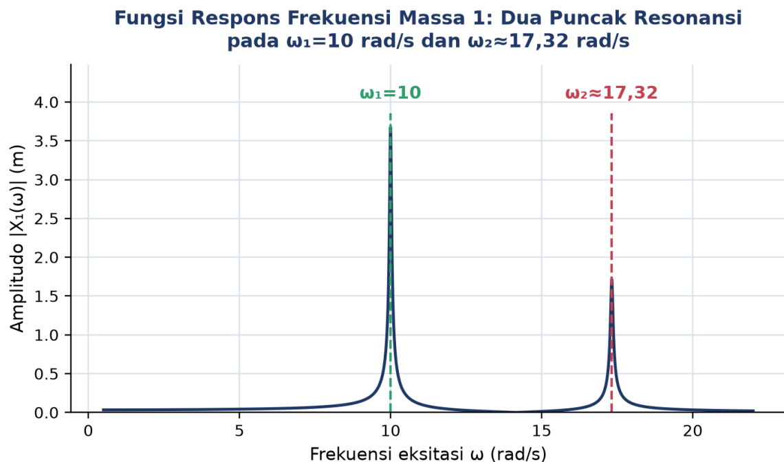
Gambar 3. Fungsi respons frekuensi amplitudo massa 1 pada sistem referensi, menunjukkan dua puncak resonansi tepat pada \omega_1=10 rad/s dan \omega_2\approx 17,32 rad/s.
