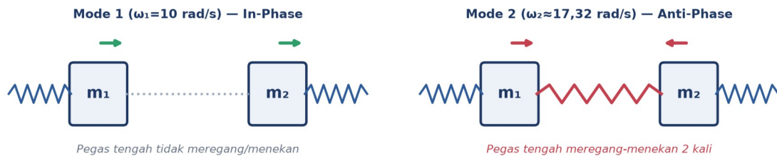
Gambar 4. Ilustrasi mode shape: Mode 1 in-phase (kedua massa bergerak searah, pegas tengah tidak bekerja) versus Mode 2 anti-phase (kedua massa berlawanan arah, pegas tengah meregang-menenakan dua kali).
