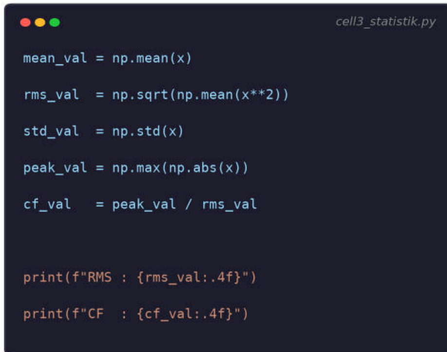
Gambar 8. Potongan Cell 3: perhitungan lima statistik dasar sinyal dengan NumPy.
