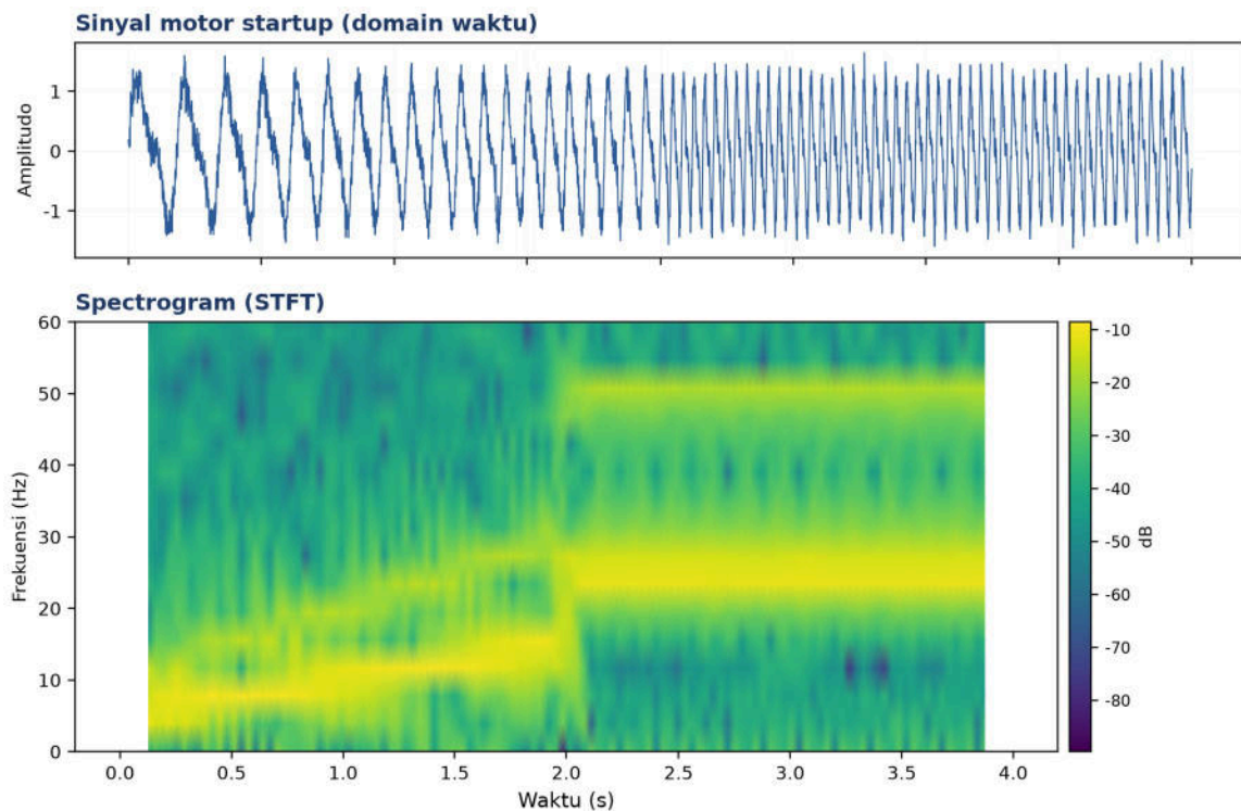
Gambar 6. Spectrogram sinyal motor startup: frekuensi dasar naik dari 5 Hz ke 25 Hz disertai harmonik kedua, terlihat jelas pada representasi waktu-frekuensi dibanding domain waktu saja.
