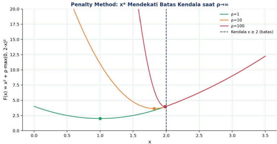
Gambar 7. Penalty method: F(x) = x^2 + \rho \cdot \max(0, 2-x)^2 untuk \rho = 1, 10, 100 ; solusi x^* semakin mendekati batas kendala x \geq 2 saat \rho membesar.
