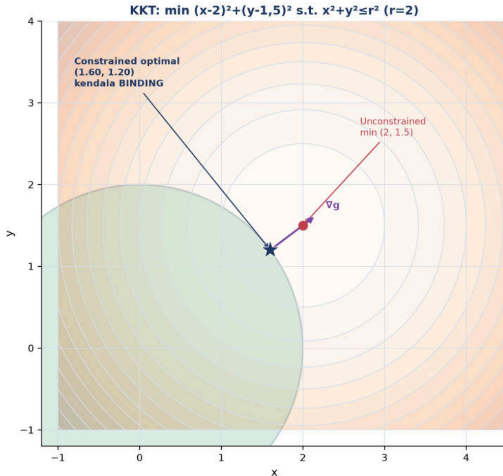
Gambar 4. Visualisasi KKT: \min (x-2)^2 + (y-1.5)^2 dengan kendala x^2 + y^2 \leq 4 ; optimal tanpa kendala (2, 1.5) berada di luar daerah feasible, sehingga solusi constrained bergeser ke batas lingkaran di mana gradien kendala \nabla g sejajar dengan arah menuju optimum tanpa kendala, sesuai kondisi stasioner KKT.
