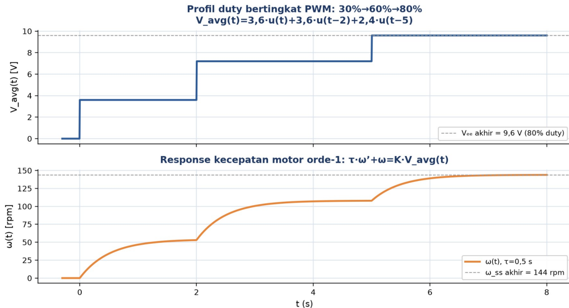
Gambar 7. Studi kasus PWM motor control: profil tegangan rata-rata V_{avg}(t) hasil tiga step duty bertingkat (panel atas) dan response kecepatan motor \omega(t) orde-1 dengan time constant \tau = 0,5 detik (panel bawah).
