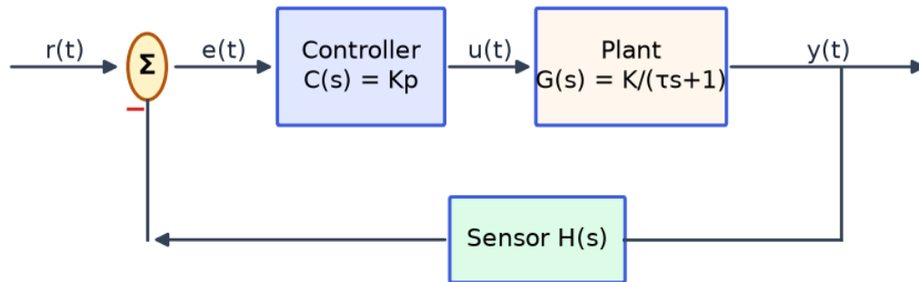
Gambar 2. Struktur baku sistem kontrol loop tertutup beserta penamaan sinyal r , e , u , dan y .
