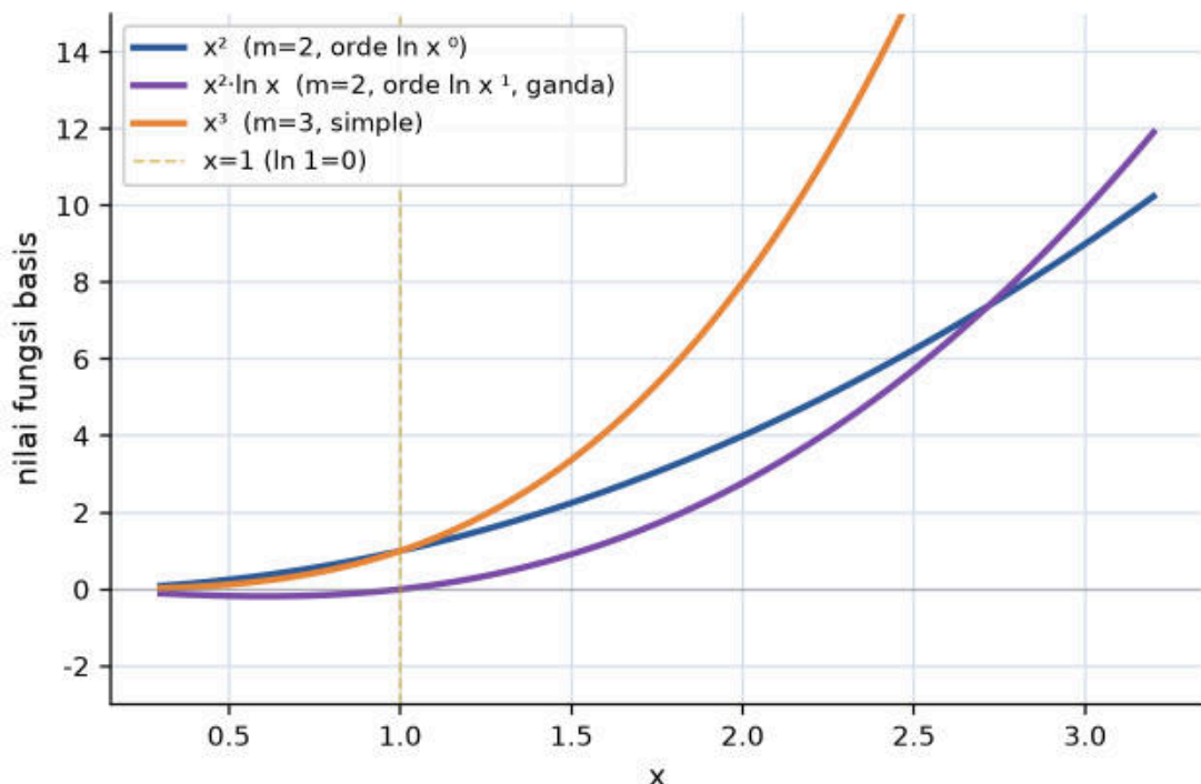
Gambar 4. Tiga fungsi basis Contoh 7.2: x^2 dan x^2 \cdot \ln x (pasangan dari akar berganda m=2 ), serta x^3 (dari akar simple m=3 ).
