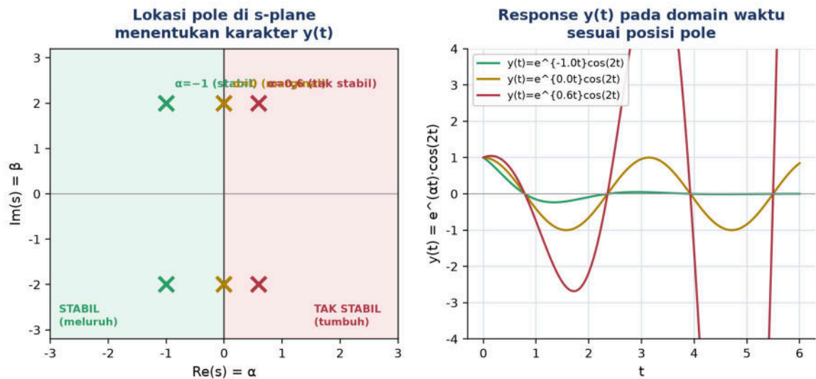
Gambar 2. Lokasi pole di s- plane menentukan karakter response y(t) : pole di kiri sumbu imajiner ( \text{Re}(s) negatif) menghasilkan peluruhan stabil, pole tepat di sumbu imajiner menghasilkan osilasi murni marginal, dan pole di kanan sumbu imajiner ( \text{Re}(s) positif) menghasilkan pertumbuhan tak stabil.
