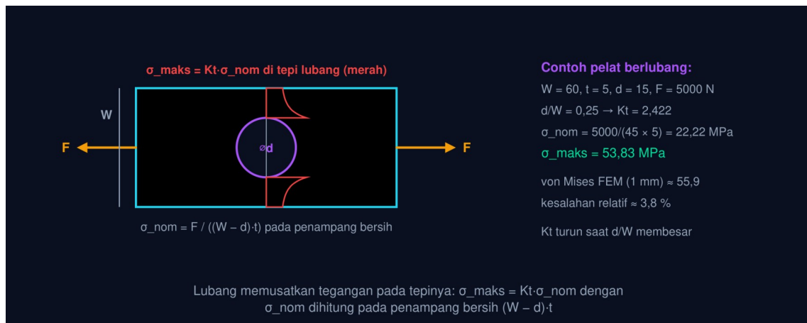
Gambar 6 — Pelat berlubang tarik: konsentrasi tegangan di tepi lubang dan tegangan nominal. Pelat W = 60, t = 5 , lubang \varnothing 15, F = 5000 \text{ N} : d/W = 0,25 memberi K_t = 2,422 ; \sigma_{\text{nom}} pada penampang bersih 22,22 \text{ MPa} , sehingga \sigma_{\text{maks}} = 53,83 \text{ MPa} di tepi lubang.
