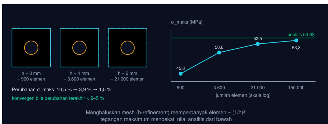
Gambar 5 — Konvergensi mesh pelat berlubang: tiga tingkat kehalusan dan grafik \sigma_{maks} terhadap jumlah elemen. Ukuran elemen 8 \rightarrow 1 mm menaikkan jumlah elemen dari \approx 900 ke \approx 150.000; \sigma_{maks} naik dari 45,8 ke 53,3 MPa mendekati nilai analitis 53,83 MPa, dengan perubahan terakhir 1,5 %.
