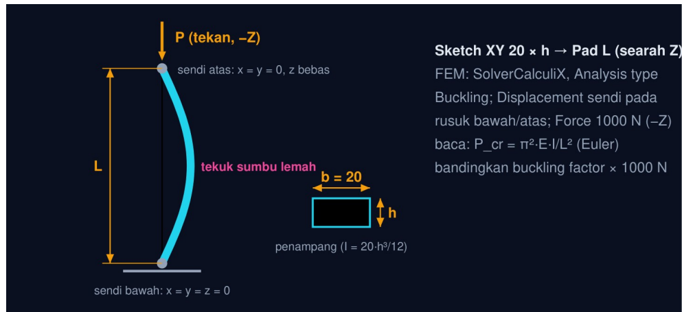
Gambar acuan: kolom sendi–sendi 20 × h: beban kritis Euler vs CalculiX Buckling. Simbol mengikuti teks tugas; angka dimensi milik Anda muncul setelah masuk.
