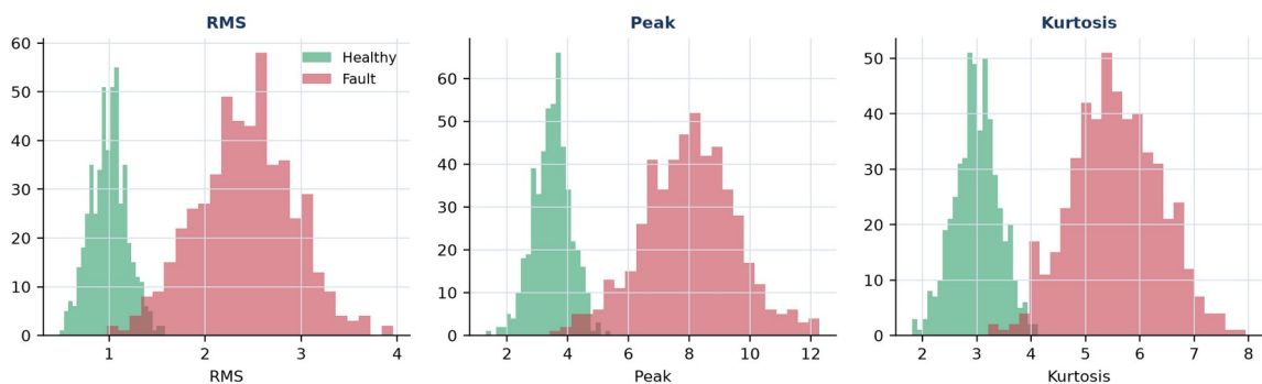
Gambar 7. Distribusi tiga fitur (RMS, Peak, Kurtosis) untuk kelas healthy vs fault pada dataset sintetis Cell 1; overlap minimal menunjukkan fitur cukup diskriminatif.
