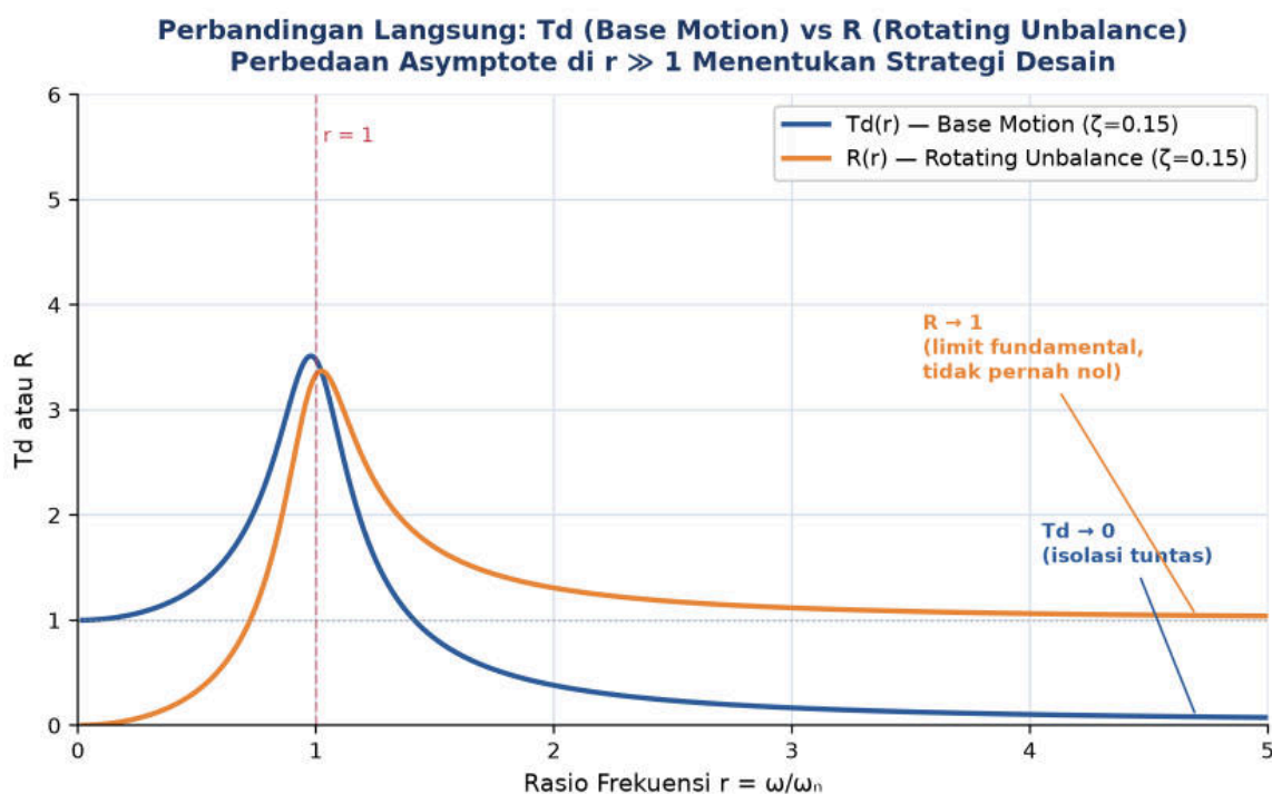
Gambar 6. Perbandingan langsung kuantitas T_d (base motion) dan R (rotating unbalance) pada \zeta yang sama, menunjukkan perbedaan asymptote di r besar.
