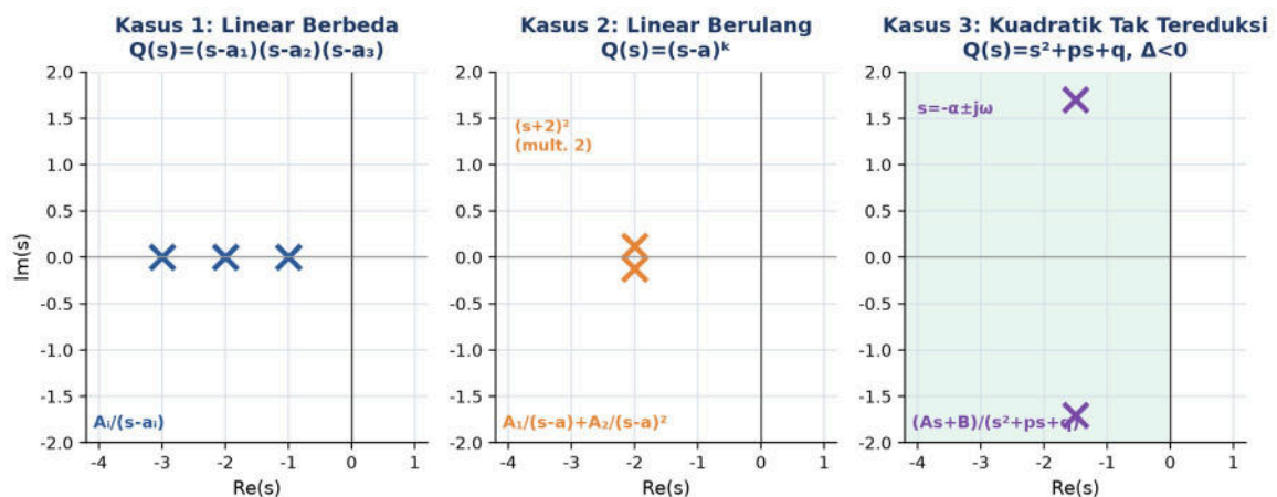
Gambar 2. Visualisasi tiga kasus faktorisasi Q(s) di s-plane: pole real berbeda (kiri), pole real berulang multiplicity 2 (tengah), dan pole kompleks konjugat dari faktor kuadratik tak tereduksi (kanan).
