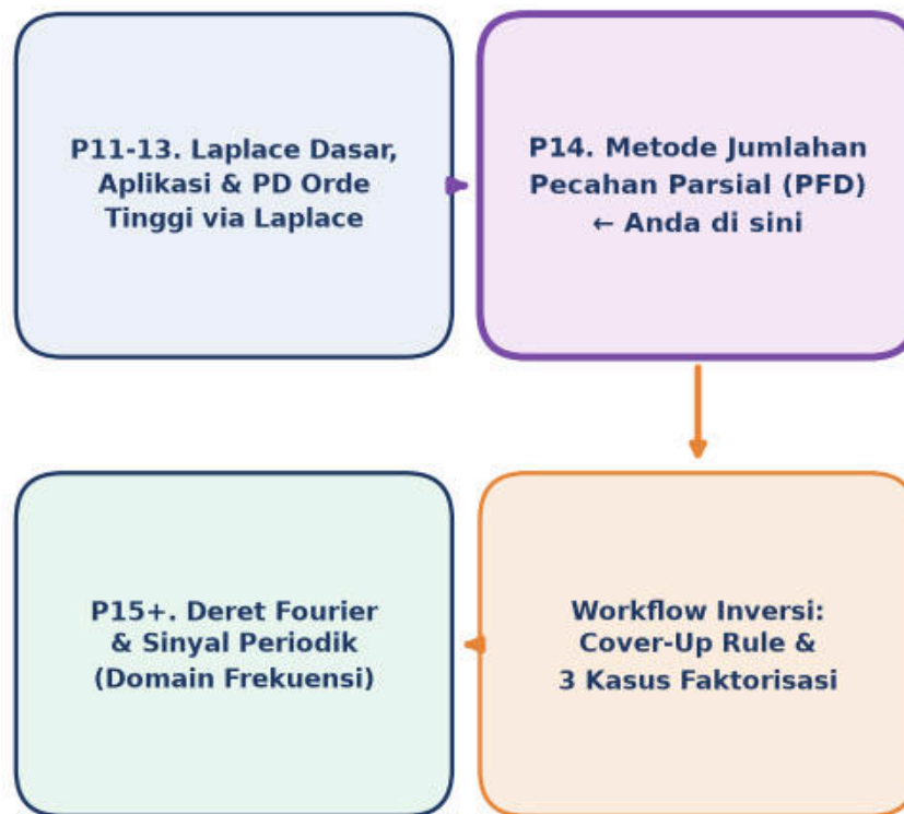
Gambar 1. Posisi Pertemuan 14 (Metode Jumlahan Pecahan Parsial) dalam alur mata kuliah Matematika 4, menjembatani tool kit Laplace dari Pertemuan 11-13 menuju ke Deret Fourier dan Pertemuan 15.
