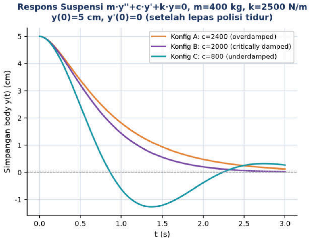
Gambar 7. Respons tiga konfigurasi suspensi m \cdot y'' + c \cdot y' + k \cdot y = 0 terhadap gangguan awal y(0)=5 cm, y'(0)=0 Konfig A (overdamped) dan B (critically damped) meluruh monoton, sedangkan Konfig C (underdamped) berosilasi melewati nol sebelum meluruh.
