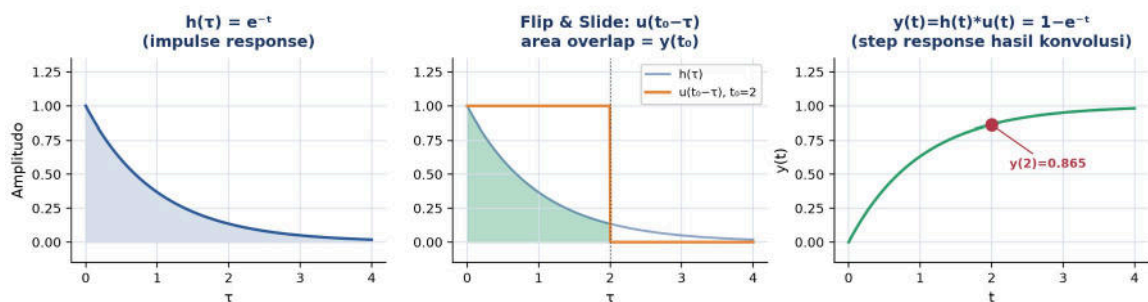
Gambar 5 | Ilustrasi sliding integral konvolusi: h(\tau)=e^{-\tau} (kiri), u(t_0-\tau) di-flip dan digeser dengan area overlap = y(t_0) (tengah), dan hasil y(t)=h(t) \cdot u(t)=1-e^{-t} sebagai step response (kanan).
