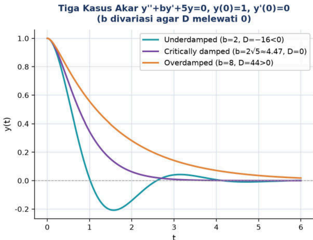
Gambar 2. Solusi y(t) dari PD y'' + b \cdot y' + 5y = 0 dengan VP y(0)=1 , y'(0)=0 untuk tiga nilai b yang mewakili tiga kasus akar ( b=2 underdamped D < 0 , b=2\sqrt{5} critically damped D=0 , b=8 overdamped D > 0 ).
