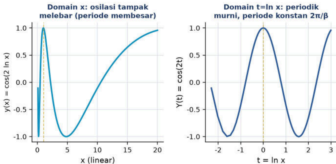
Gambar 5 Ef eks substitusi t = \ln x pada Contoh 6.3: domain x menampilkan osilasi yang tampak melebar, domain t = \ln x menampilkan osilasi periodik murni dengan periode konstan.
