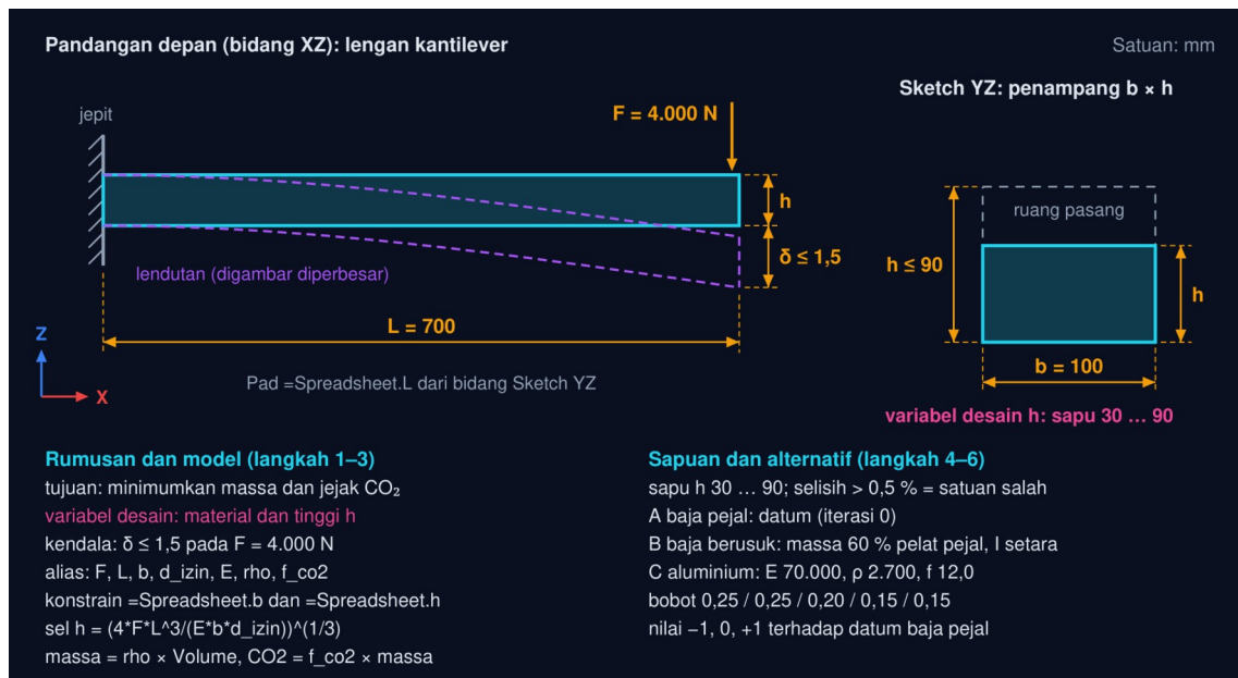
Gambar 7 — Gambar kerja lengan braket kantilever dengan variabel desain h . Ukuran dalam mm, gaya dalam N. Lengan pejal b \times h \times L dijepit pada bidang Sketch YZ dan memikul F = 4.000 N di ujung bebas dengan kendala lendutan ujung \delta \leq 1,5 (langkah 1); penampangnya adalah sketsa b \times h pada langkah 2. Tinggi h adalah variabel desain: dihitung dari kendala pada langkah 3, disapu 30–90 pada langkah 4, dan dibatasi ruang pasang h \leq 90 . Catatan memuat alias, rumus, dan angka alternatif yang diketik pada langkah 1–6.
