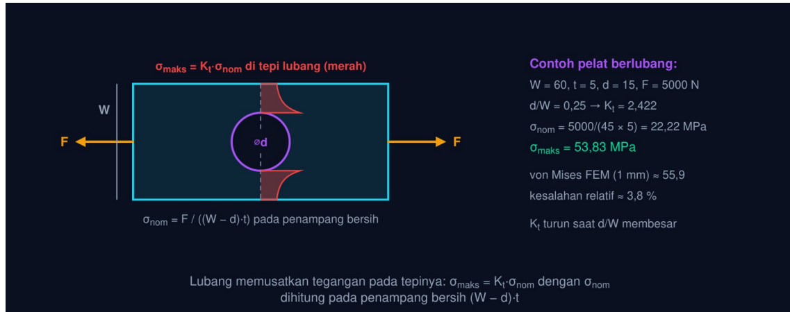
Gambar 6 — Pelat berlubang tarik: konsentrasi tegangan di tepi lubang dan tegangan nominal. Pelat W = 60 , t = 5 , lubang \varnothing 15 , F = 5000 \text{ N} : d/W = 0,25 memberi K_t = 2,422 ; \sigma_{nom} pada penampang bersih 22,22 \text{ MPa} , sehingga \sigma_{maks} = 53,83 \text{ MPa} di tepi lubang.
