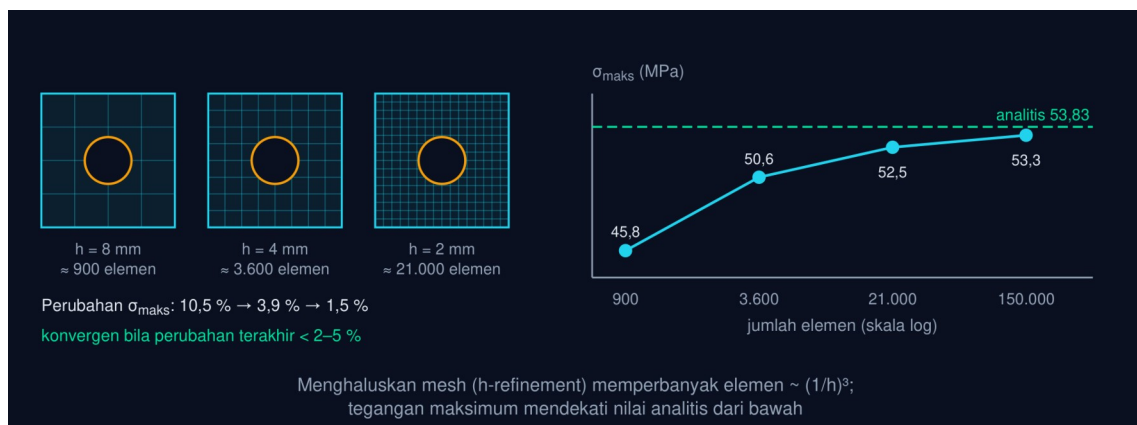
Gambar 5 — Konvergensi mesh pelat berlubang: tiga tingkat kehalusan dan grafik \sigma_{maks} terhadap jumlah elemen. Ukuran elemen 8 \rightarrow 1 mm menaikkan jumlah elemen dari \approx 900 ke \approx 150.000; \sigma_{maks} naik dari 45,8 ke 53,3 MPa mendekati nilai analitis 53,83 MPa, dengan perubahan terakhir 1,5 %.
