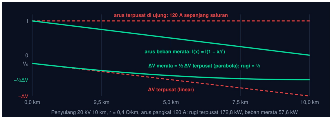
Gambar 5 — Arus, tegangan, dan rugi sepanjang penyulang: beban terpusat vs tersebar merata. Bila beban terpusat di ujung, arus sama sepanjang saluran dan tegangan turun linear; bila tersebar merata, arus berkurang linear sehingga tegangan turun parabolik dengan jatuh total setengahnya dan rugi sepertiganya: 172,8 → 57,6 kW pada penyulang contoh.
