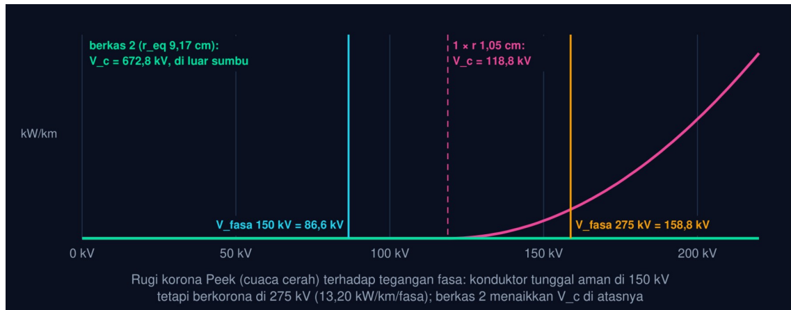
Gambar 6 — Tegangan kritis korona dan rugi korona: konduktor tunggal vs berkas. Konduktor tunggal r = 1,05 cm berkorona di atas 119 kV fasa: aman pada 150 kV, tetapi pada 275 kV membuang 13,2 kW/km/fasa. Berkas dua sub-konduktor menaikkan tegangan kritis ke 673 kV.
