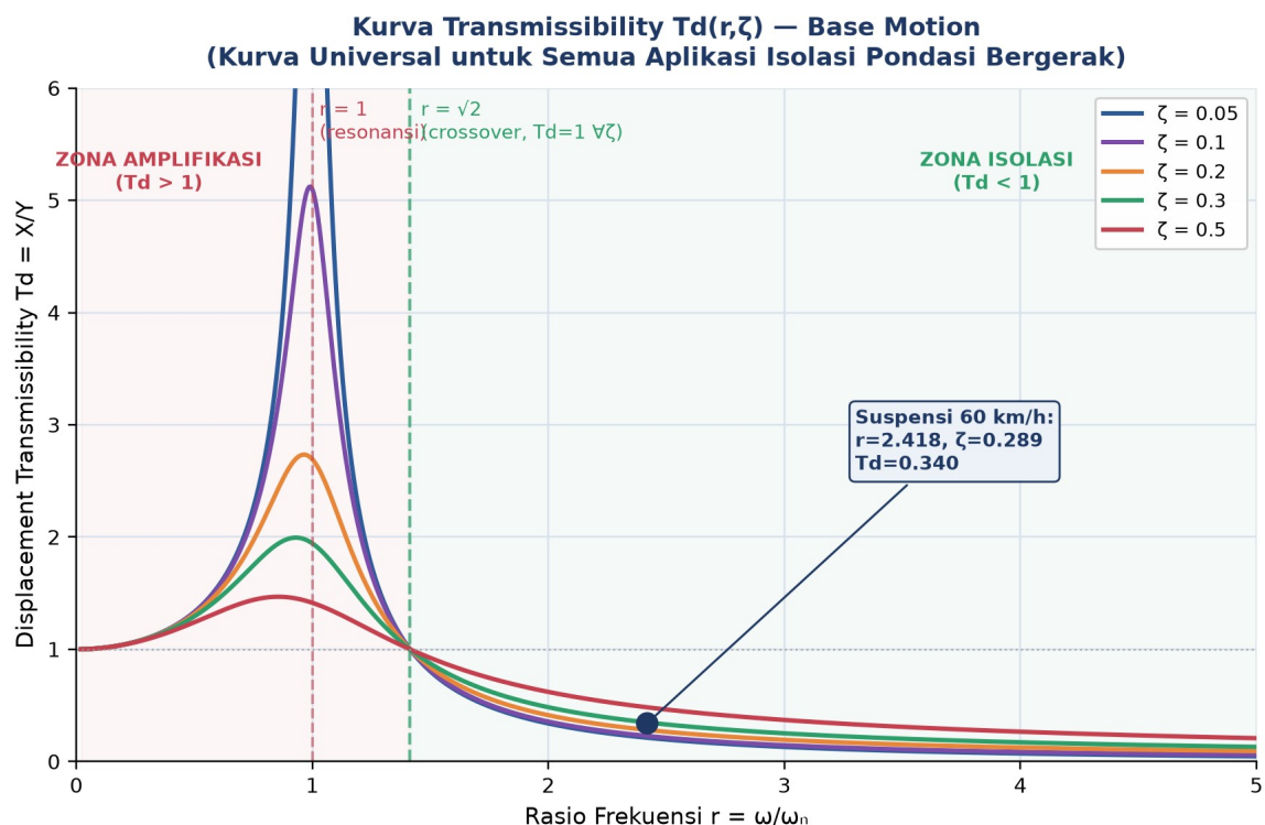
Gambar 3. Kurva transmissibility T_d(r, \zeta) untuk lima nilai \zeta , dengan crossover r=\sqrt{2} dan marker contoh suspensi mobil pada 60 km/jam.
