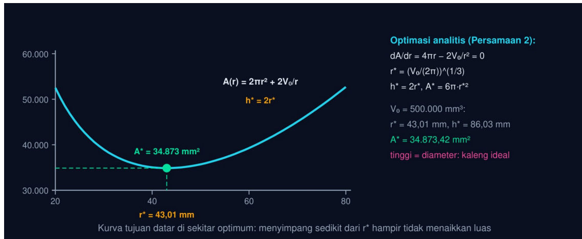
Gambar 4 — Kaleng tertutup dengan luas permukaan minimum. Untuk volume tetap 500.000 mm³, luas A(r) = 2\pi r^2 + 2V_0/r mencapai minimum 34.873,42 mm² pada r^* = 43,01 mm dengan h^* = 2r^* = 86,03 mm — tinggi persis sama dengan diameter.
