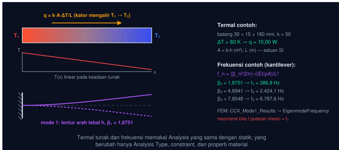
Gambar 6 — Hantaran kalor batang dan mode getar pertama kantilever. Batang 30 × 15 × 180 mm dengan \Delta T = 80 \text{ K} menghantarkan q = 10,00 \text{ W} ( k = 50 ); kantilever yang sama bergetar pada f_1 = 386,8 \text{ Hz} , f_2 = 2.424,1 \text{ Hz} , f_3 = 6.787,6 \text{ Hz} .
