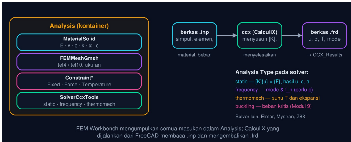
Gambar 2 — Objek FEM Workbench di dalam Analysis dan jalur solver CalculiX. Material, mesh, constraint, dan solver hidup di dalam kontainer Analysis; saat dijalankan, FreeCAD menulis .inp, memanggil ccx, dan membaca .frd menjadi CCX_Results.
