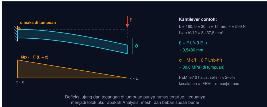
Gambar 5 — Kantilever terdefleksi, diagram momen, dan rumus validasi \delta dan \sigma . Kantilever 180 \times 30 \times 15 \text{ mm} baja dengan F = 500 \text{ N} : \delta = 0,5486 \text{ mm} dan \sigma \text{ maks} = 80,0 \text{ MPa} di tumpuan; FEM tet10 halus harus mendekati keduanya.
