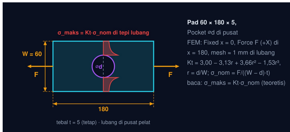
▲ Gambar acuan: pelat berlubang tarik: konsentrasi tegangan Kt \cdot \sigma_{nom} vs von Mises FEM. Simbol mengikuti teks tugas; angka dimensi milik Anda muncul setelah masuk.
