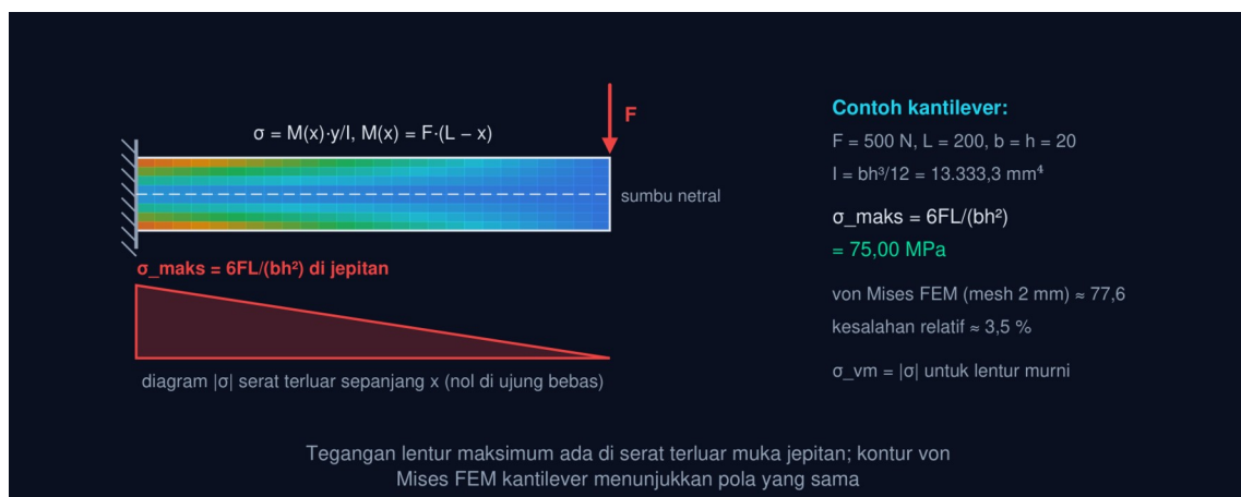
Gambar 2 — Distribusi tegangan lentur kantilever dan kontur von Mises. Kantilever 20 \times 20 \text{ mm} , L = 200 \text{ mm} , F = 500 \text{ N} : tegangan lentur terbesar di serat terluar muka jepitan, \sigma_{maks} = 6FL/(bh^2) = 75,00 \text{ MPa} ; kontur von Mises FEM menampilkan pola merah di jepitan yang memudar ke ujung bebas.
