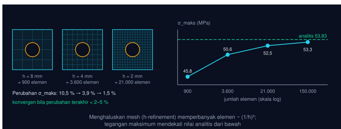
Gambar 5 — Konvergensi mesh pelat berlubang: tiga tingkat kehalusan dan grafik \sigma_{maks} terhadap jumlah elemen. Ukuran elemen 8 \rightarrow 1 \text{ mm} menaikkan jumlah elemen dari \approx 900 ke \approx 150.000 ; \sigma_{maks} naik dari 45,8 ke 53,3 MPa mendekati nilai analitis 53,83 MPa, dengan perubahan terakhir 1,5 %.
