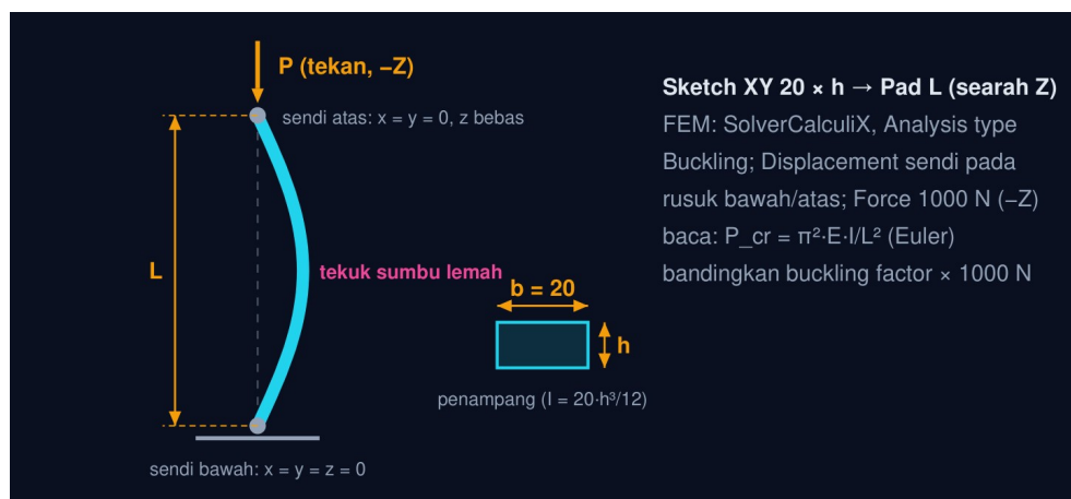
▲ Gambar acuan: kolom sendi–sendi 20 \times h : beban kritis Euler vs CalculiX Buckling. Simbol mengikuti teks tugas; angka dimensi milik Anda muncul setelah masuk.
