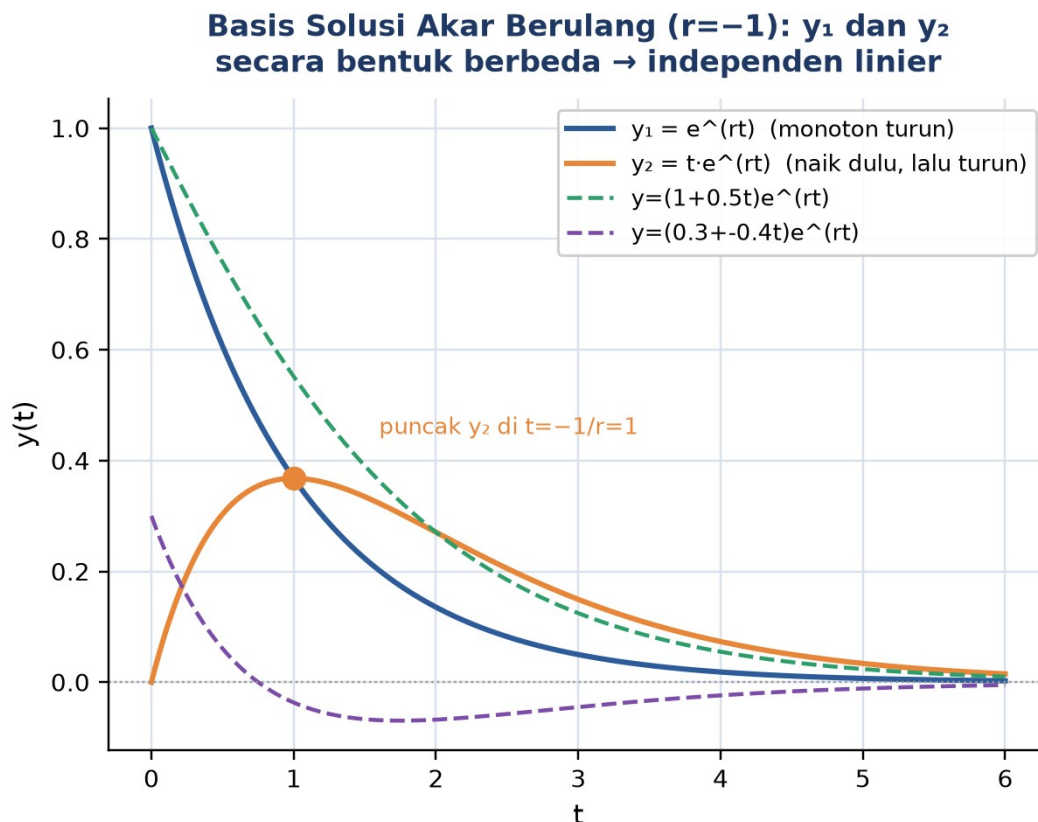
Gambar 4. Basis solusi akar berulang r=-1 : y_1=e^{(rx)} monoton turun sejak awal, sedangkan y_2=x \cdot e^{(rx)} naik dahulu mencapai puncak di x=-1/r lalu turun; kombinasi (C_1+C_2x)e^{(rx)} untuk berbagai C_1, C_2 menghasilkan bentuk kurva yang beragam.
