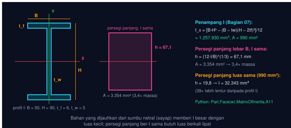
Gambar 6 — Penampang I versus persegi panjang dengan momen inersia sama. Profil I B = 50, H = 90, t f = 6, t w = 5 memiliki I x = 1.257.930 mm 4 dengan luas 990 mm 2 ; persegi panjang selebar B yang sama kakunya harus setinggi 67,1 mm dengan luas 3.354 mm 2 , 3,4 kali massa.
