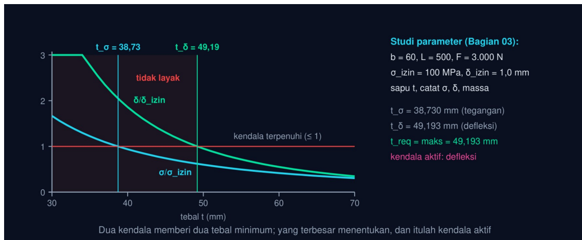
Gambar 3 — Studi parameter tebal pelat dengan dua kendala. Pelat kantilever baja 60 mm × t × 500 mm memikul 3.000 N: kendala tegangan menuntut t \geq 38,730 mm dan kendala defleksi menuntut t \geq 49,193 mm; daerah merah tidak layak, sehingga t_{req} = 49,193 mm dengan kendala defleksi sebagai kendala aktif.
