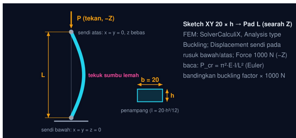
▲ Gambar acuan: kolom sendi–sendi 20 × h: beban kritis Euler vs CalculiX Buckling. Simbol mengikuti teks tugas; angka dimensi milik Anda muncul setelah masuk.
