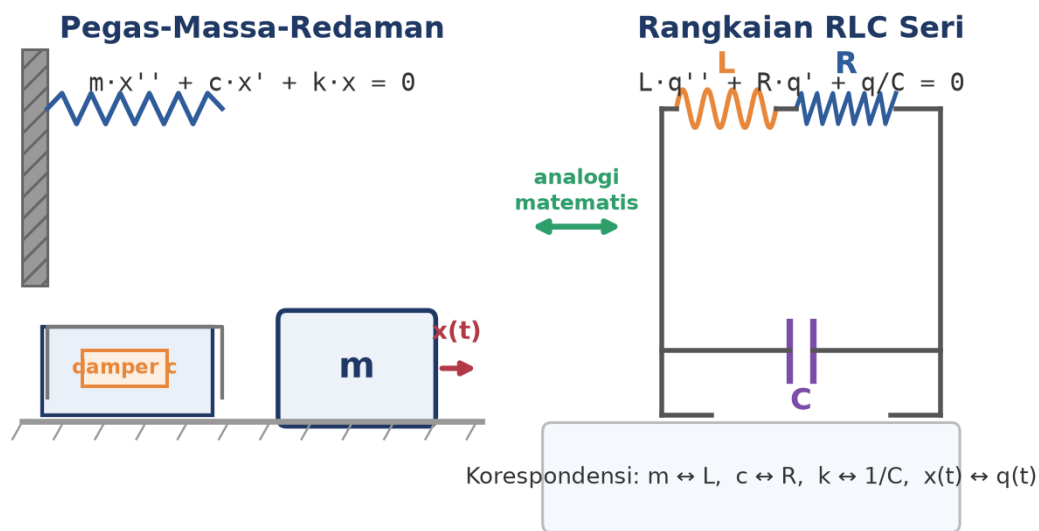
Gambar 6. Analogi mekanik-listrik: sistem pegas-massa-redaman m \cdot x'' + c \cdot x' + k \cdot x = 0 (kiri) identik secara matematis dengan rangkaian RLC seri L \cdot q'' + R \cdot q' + q/C = 0 (kanan), dengan korespondensi m \leftrightarrow L , c \leftrightarrow R , k \leftrightarrow 1/C .
