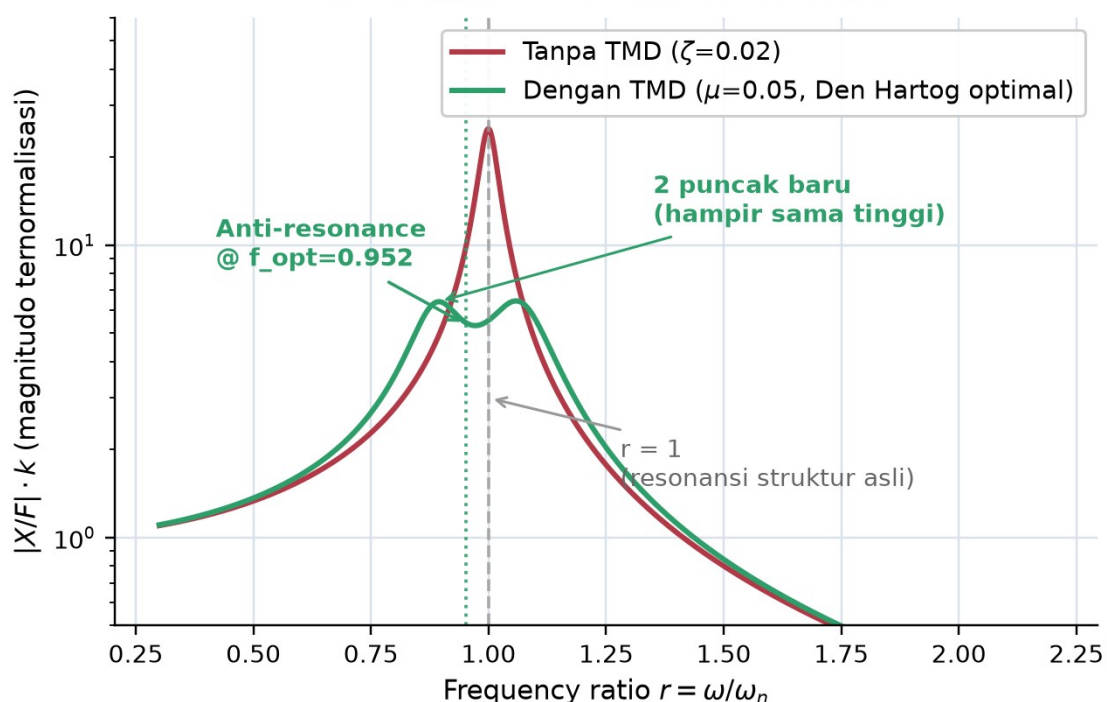
Gambar 3. FRF struktur utama tanpa TMD (satu puncak tajam di r=1 ) dibandingkan dengan TMD optimal Den Hartog \mu=0,05 (anti-resonance dangkal dan dua puncak baru hampir sama tinggi), sistem referensi m=1 kg, k=100 N/m, \omega_n=10 rad/s.
