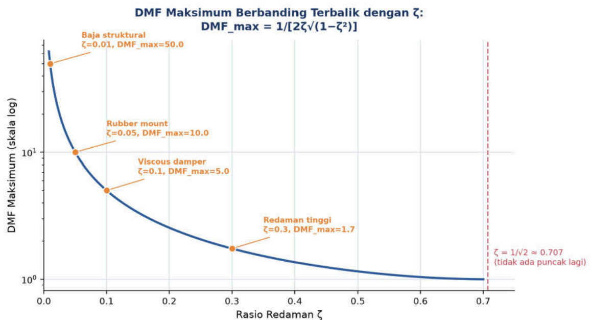
Gambar 3 Hubungan DMF_{\text{maksimum}} terhadap rasio redaman \zeta (skala log aritmik), menunjukkan sifat berbanding terbalik yang tajam.
