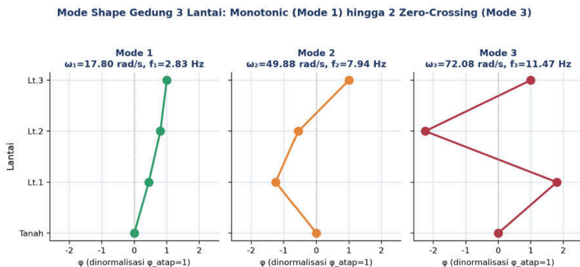
Gambar 4. Mode shape gedung 3 lantai: Mode 1 monotonic (0 zero crossing), Mode 2 dengan 1 zero crossing, Mode 3 dengan 2 zero crossing.
