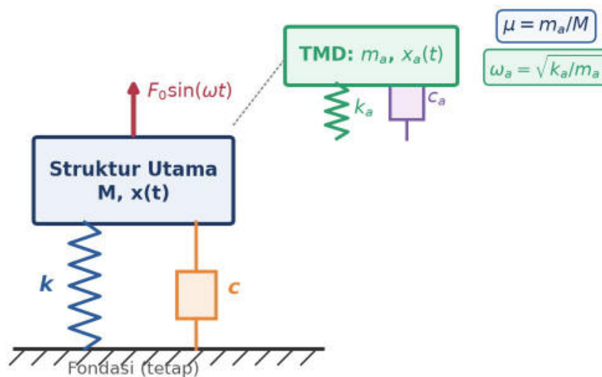
Gambar 2 Skematik TMD terpasang pada struktur utama: massa M dengan pegas k dan damper c menerima eksitasi F_0 \sin(\omega t) , TMD (massa m_a , pegas k_a , dan damper c_a ) terpasang pada M sebagai sistem massa-pegas-damper auxiliary.
