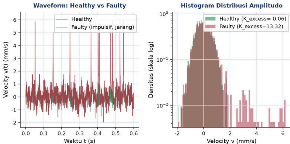
Gambar 4. Histogram distribusi amplitudo (skala log): sinyal mendekati Gaussian (excess kurtosis kira-kira nol) versus sinyal dengan spike jarang amplitudo besar (excess kurtosis jauh di atas nol, ekor distribusi memanjang).
