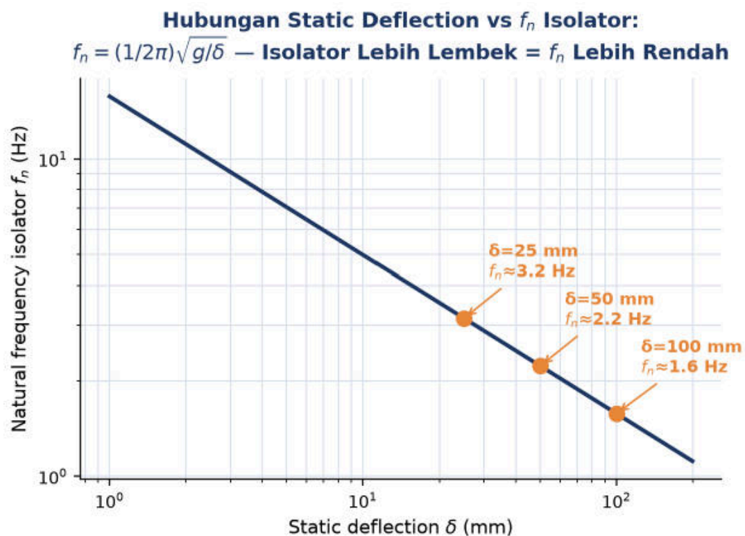
Gambar 6. Hubungan static deflection \delta terhadap natural frequency isolator f_n , menunjukkan bahwa isolator yang lebih lembek ( \delta besar) menghasilkan f_n lebih rendah, ditandaikan tiga titik acuan praktis \delta = 25, 50 dan 100 mm.
