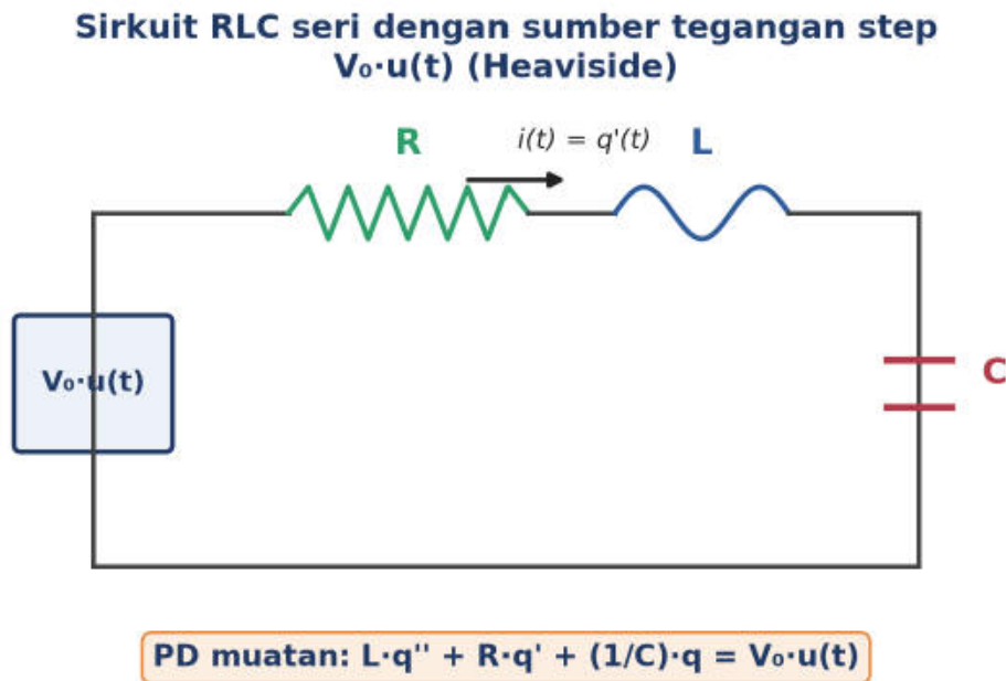
Gambar 6 Skema sirkuit RLC seri dengan sumber tegangan step V_0 u(t) (Heaviside), memodelkan PD muatan L \cdot q'' + R \cdot q' + (1/C) \cdot q = V_0 u(t) .
