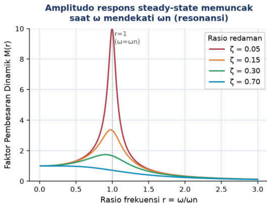
Gambar 6 . Faktor Pembesaran Dinamik (Dynamic Magnification Factor) M(r) terhadap rasio frekuensi r = \omega / \omega_n untuk empat rasio redaman \zeta berbeda; puncak kurva pada r=1 menandai resonansi.
