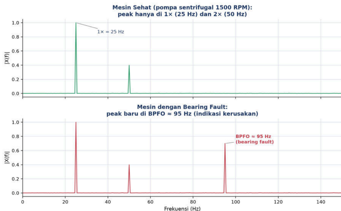
Gambar 6. Perbandingan spektrum FFT getaran pompa sentrifugal 1500 RPM: mesin sehat hanya menunjukkan peak di 1 \times dan 2 \times RPM (25 Hz dan 50 Hz), sedangkan mesin dengan bearing fault menunjukkan peak tambahan di BPFO sekitar 95 Hz.
