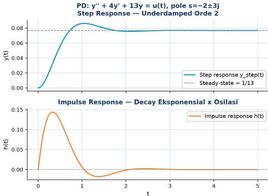
Gambar 8. Step response dan impulse response sistem orde dua underdamped dengan pole s = -2 \pm 3j , direproduksi dari Cell 4, konsistensi dengan studi kasus sirkuit RLC pada bagian aplikasi industri.
