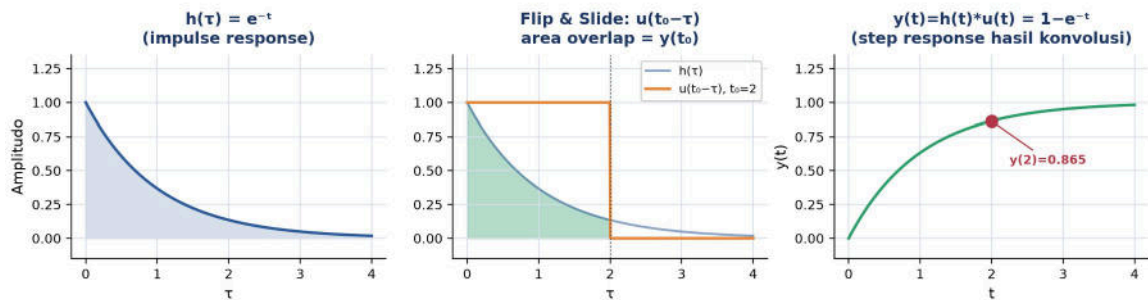
Gambar 5. Ilustrasi sliding integral konvolusi: h(\tau) = e^{-\tau} (kiri), u(t-\tau) di-flip dan digeser dengan area overlap = y(t_0) (tengah), dan hasil y(t) = h(t)*u(t) = 1 - e^{-t} sebagai step response (kanan).
