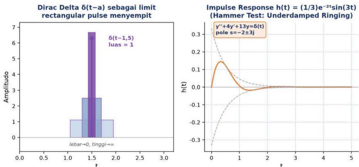
Gambar 3. Dirac delta \delta(t-1,5) sebagai limit rectangular pulse yang menyempit dengan luas tetap 1 (kiri) dan impulse response h(t) = (1/3)e^{(-2t)}\sin(3t) hasil hammer test pada sistem underdamped (kanan).
