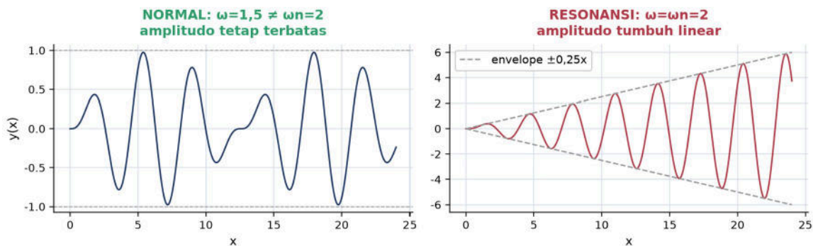
Gambar 4. Perbandingan solusi PD tanpa redaman y'' + 4y = \sin(\omega x) : panel kiri ( \omega=1,5 \neq \omega_n=2 ) amplitudo tetap terbatas; panel kanan ( \omega=\omega_n=2 , resonansi) amplitudo tumbuh linear dengan selubung \pm 0,25x .
