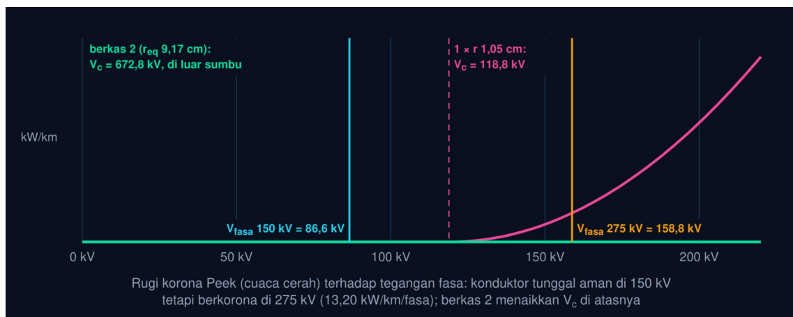
Gambar 6 — Tegangan kritis korona dan rugi korona: konduktor tunggal vs berkas. Konduktor tunggal r = 1,05 cm berkorona di atas 119 kV fasa: aman pada 150 kV, tetapi pada 275 kV membuang 13,2 kW/km/fasa. Berkas dua sub-konduktor menaikkan tegangan kritis ke 673 kV.
