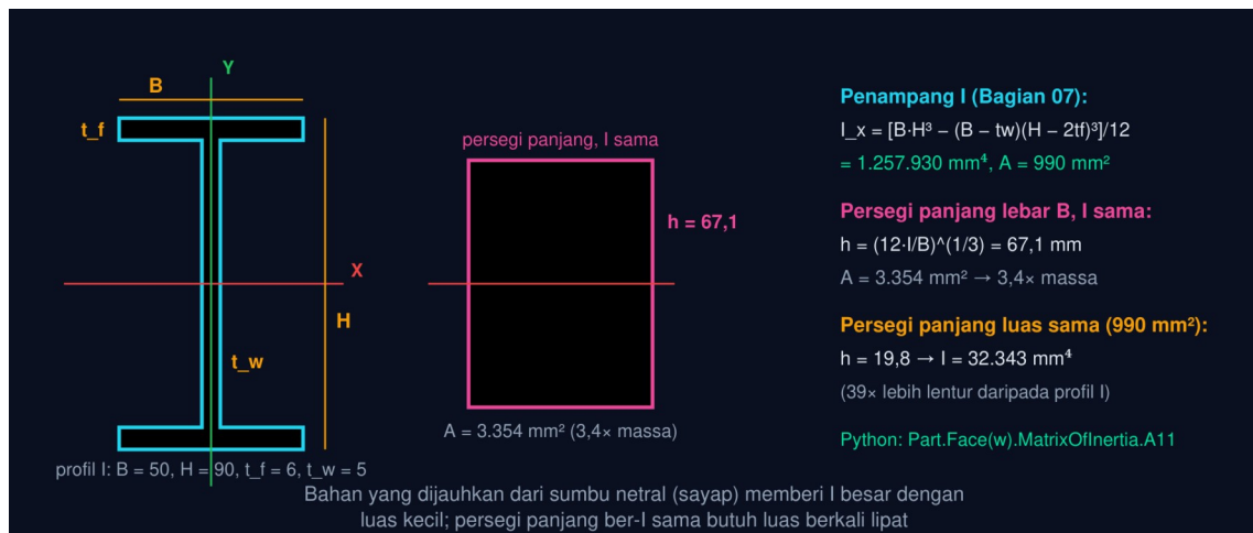
Gambar 6 — Penampang I versus persegi panjang dengan momen inersia sama. Profil I B = 50, H = 90, t_f = 6 , t_w = 5 memiliki I_x = 1.257.930 \text{ mm}^4 dengan luas 990 \text{ mm}^2 ; persegi panjang selebar B yang sama kakunya harus setinggi 67,1 mm dengan luas 3.354 \text{ mm}^2 , 3,4 kali massa.
