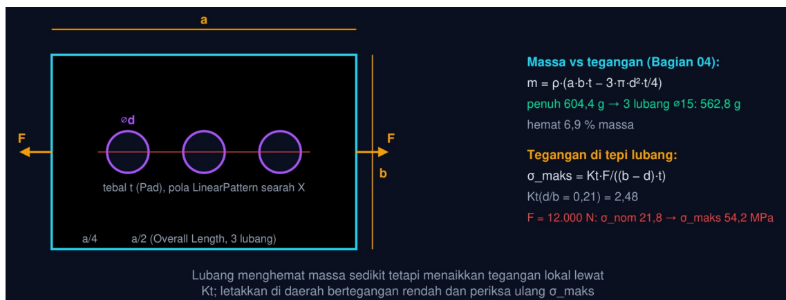
Gambar 4 — Pelat tiga lubang: massa turun, tegangan lokal naik. Pelat 110 × 70 × 10 baja (604,4 g) diberi tiga lubang \phi 15 pola linear: massa menjadi 562,8 g (hemat 6,9 %), tetapi pada beban tarik 12.000 N tegangan di tepi lubang 54,2 MPa, 2,48× tegangan nominal.
