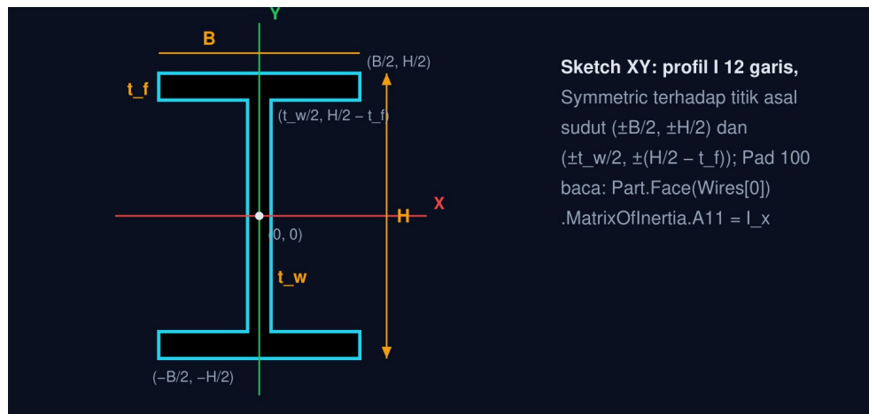
Gambar acuan: profil I simetris berpusat di titik asal dan momen inersia I_x . Simbol mengikuti teks tugas; angka dimensi milik Anda muncul setelah masuk.
