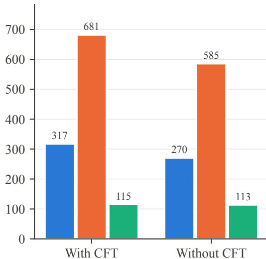
Prove (rapidsnark)
