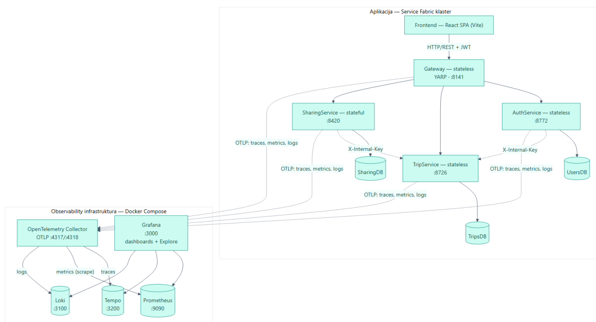
Слика 5.1. ТО-BE архитектура — додат observability слој
