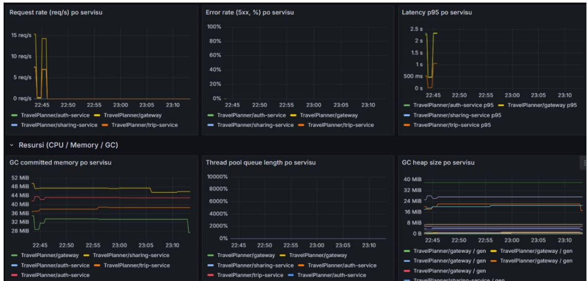
Слика 5.3. Grafana dashboard „Travel Planner - Overview”
