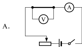
测定一段电阻丝（约 5\ \Omega ）的电阻
