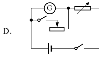
测定电流表内阻
