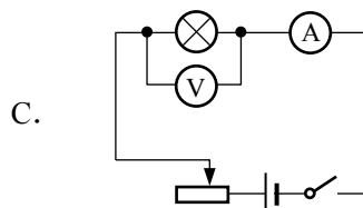
描绘小灯泡（额定电压为 2.5\ \text{V} ）的伏安特性曲线
