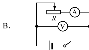
测定电源的电动势和内电阻（约 3\ \Omega ）
