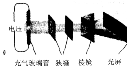
D. 氢原子发射的光经三棱镜分光后 呈现线状光谱
