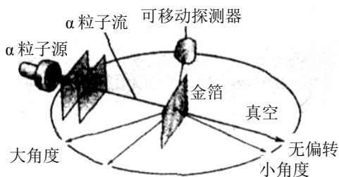
C. 轰击金箔的 \alpha 粒子中有少数运动方向发生较大偏转
