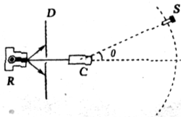
A. X 射线被石墨散射后部分波长增大
