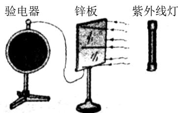
B. 锌板被紫外线照射时有电子逸出 但被可见光照射时没有电子逸出
