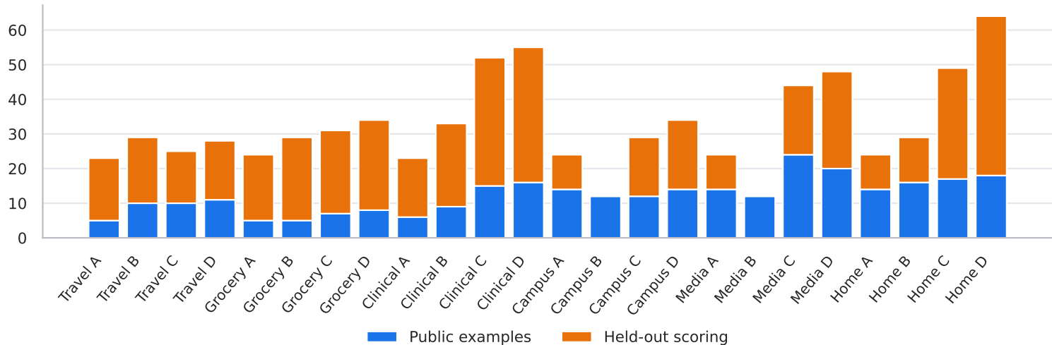
Scenario count
