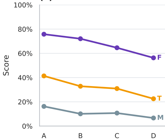
(a) Scenario-level
