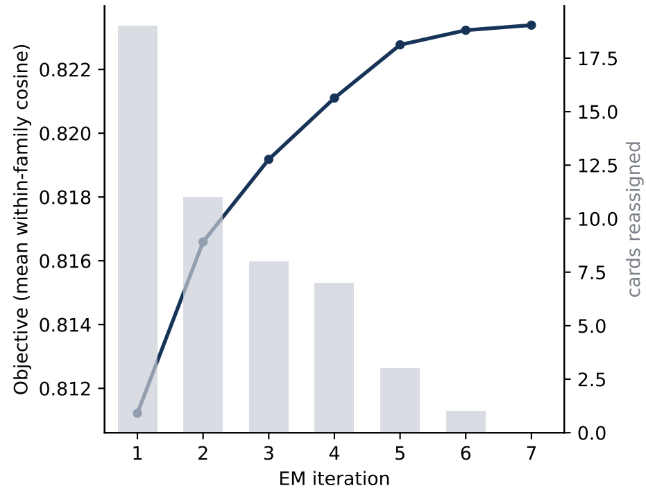
(A) EM convergence
