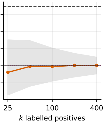
DV→BV
