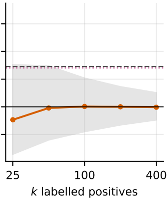
BV→DV
