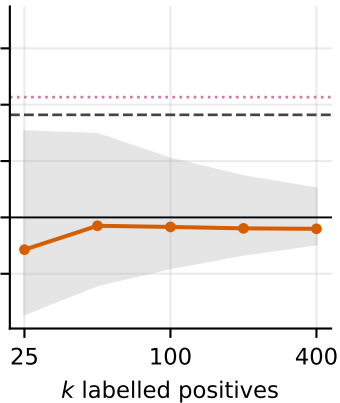
BV temporal
