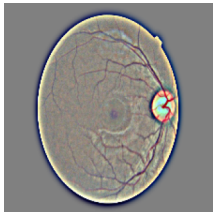
No DR (n=1805)
