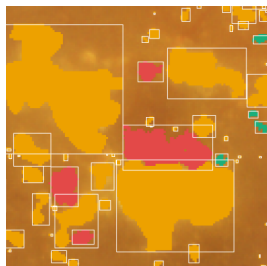
Zoom + boxes
