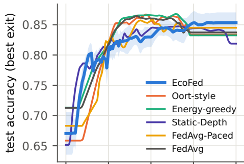
PAMAP2, \phi = 0.1
