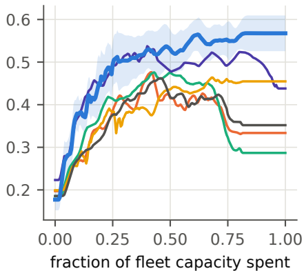
PAMAP2, \phi = 0.25
