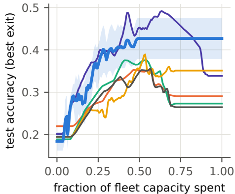
PAMAP2, \phi = 0.1
