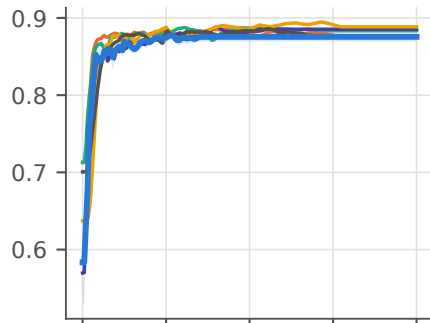
PAMAP2, \phi = 1.0
