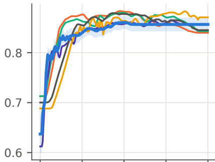
PAMAP2, \phi = 0.25
