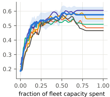
PAMAP2, \phi = 1.0
