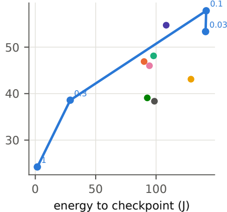
PAMAP2, \phi = 1.0
