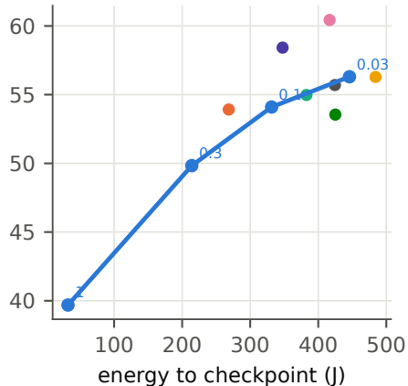
PAMAP2, \phi = 1.0
