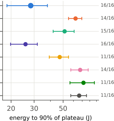
PAMAP2, \phi = 1.0
