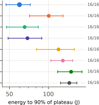
PAMAP2, \phi = 1.0
