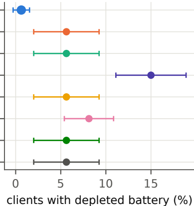
PAMAP2, \phi = 0.25
