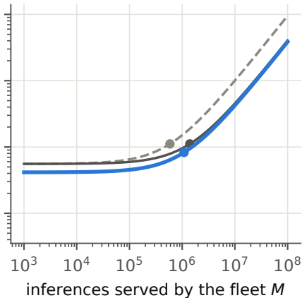
PAMAP2, \phi = 1
