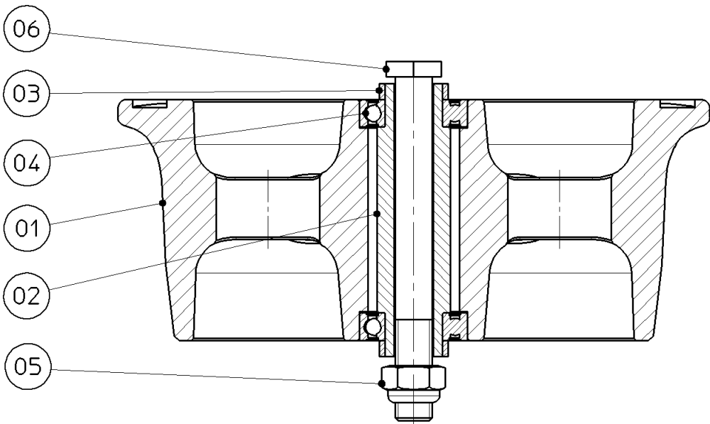
Schnitt A-A
