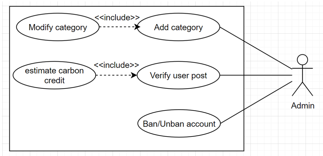
รูปที่ 22 Use Case Diagram ของ Admin ที่สามารถทำได้เพิ่มเติมจาก ผู้ใช้
