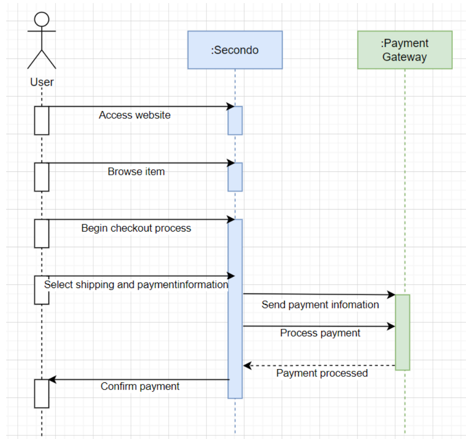
รูปที่ 23 Sequence Diagram ของการซื้อสินค้าของผู้ใช้งาน
