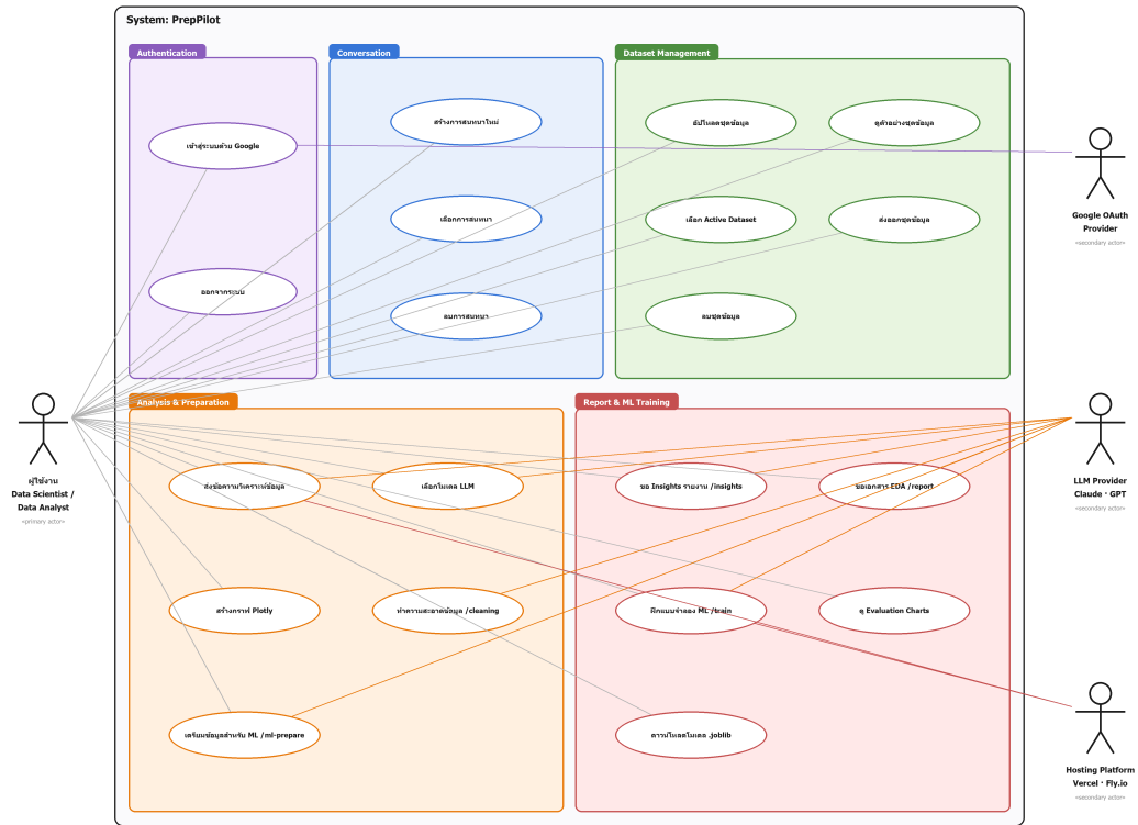
รูปที่ 3.2 Use Case Diagram ของระบบ PrepPilot
