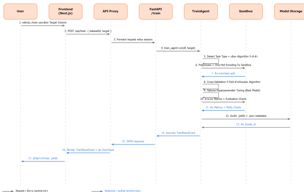
รูปที่ 3.4 Sequence Diagram ของวงจรการฝึกแบบจำลอง /train
