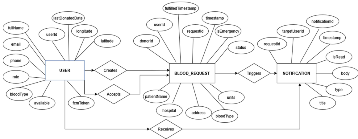
Figure 5 ER Diagram
